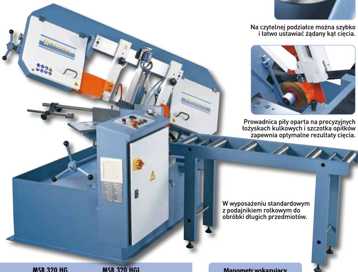
Ramie pily precyzyjnie opuszcza się za pomocą siłownika hydraulicznego.
