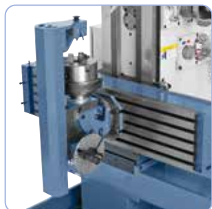
Głowica podziałowa (opcjonalna) może być używana w pozycji poziomej i pionowej.
