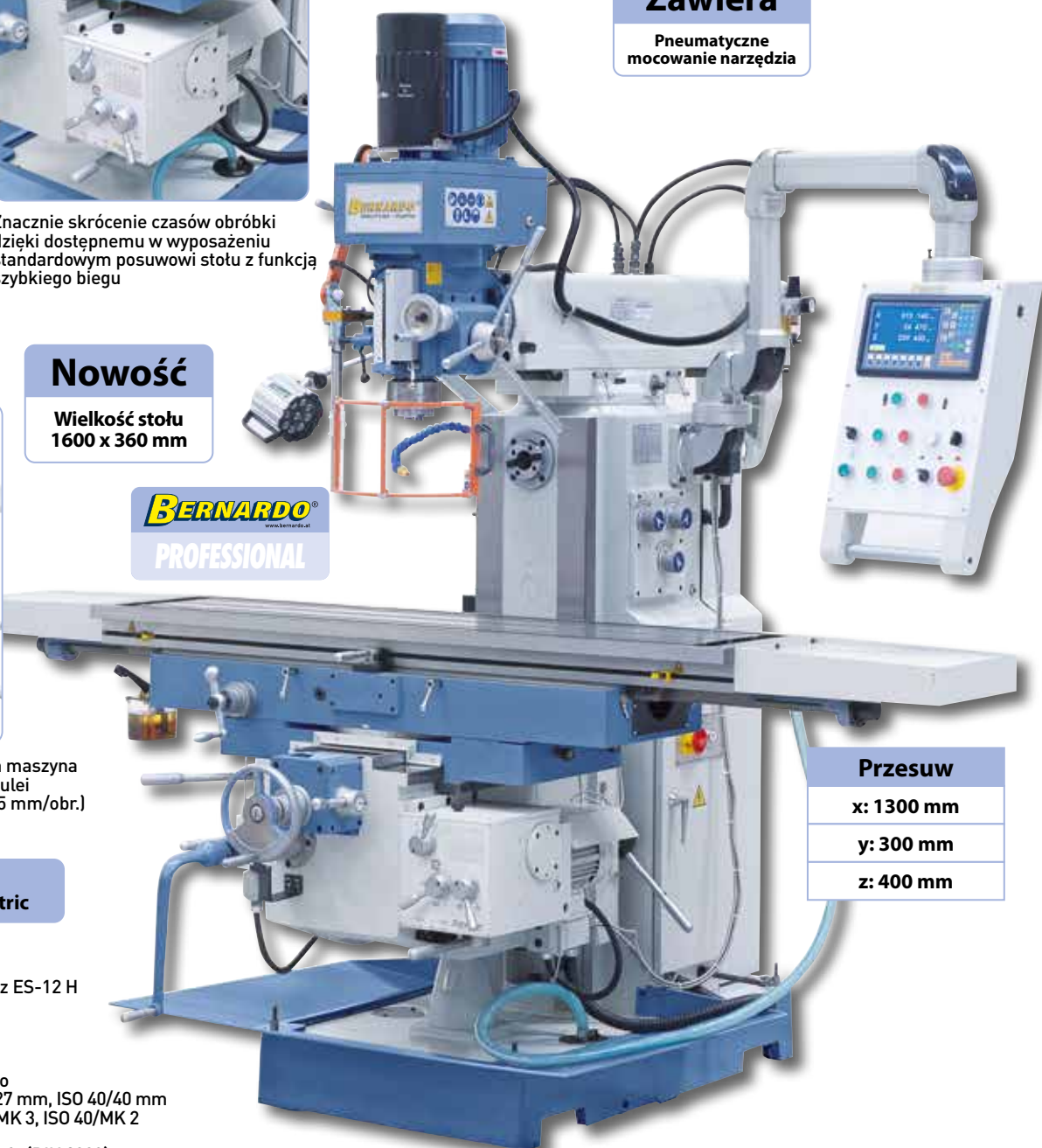
Przejrzysty panel sterujący. Wyświetlacz cyfrowy w standardzie.
