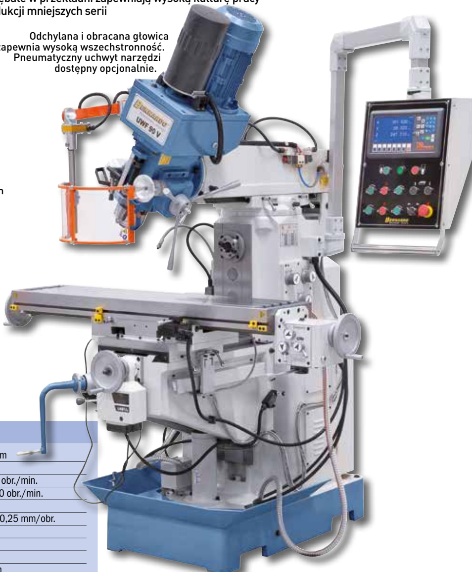
W wyposażeniu standardowym z podtrzyma i długim trzpieniem frezowym do frezowania poziomego
