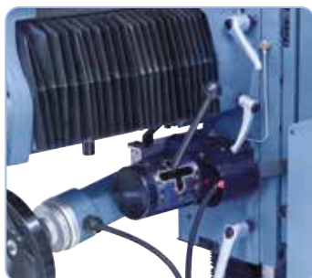
Dźwignia selektora do posuwu (rys. Oś x i z), regulacja prędkości posuwu za pomocą potencjometru z kontrolą na panelu sterowania
