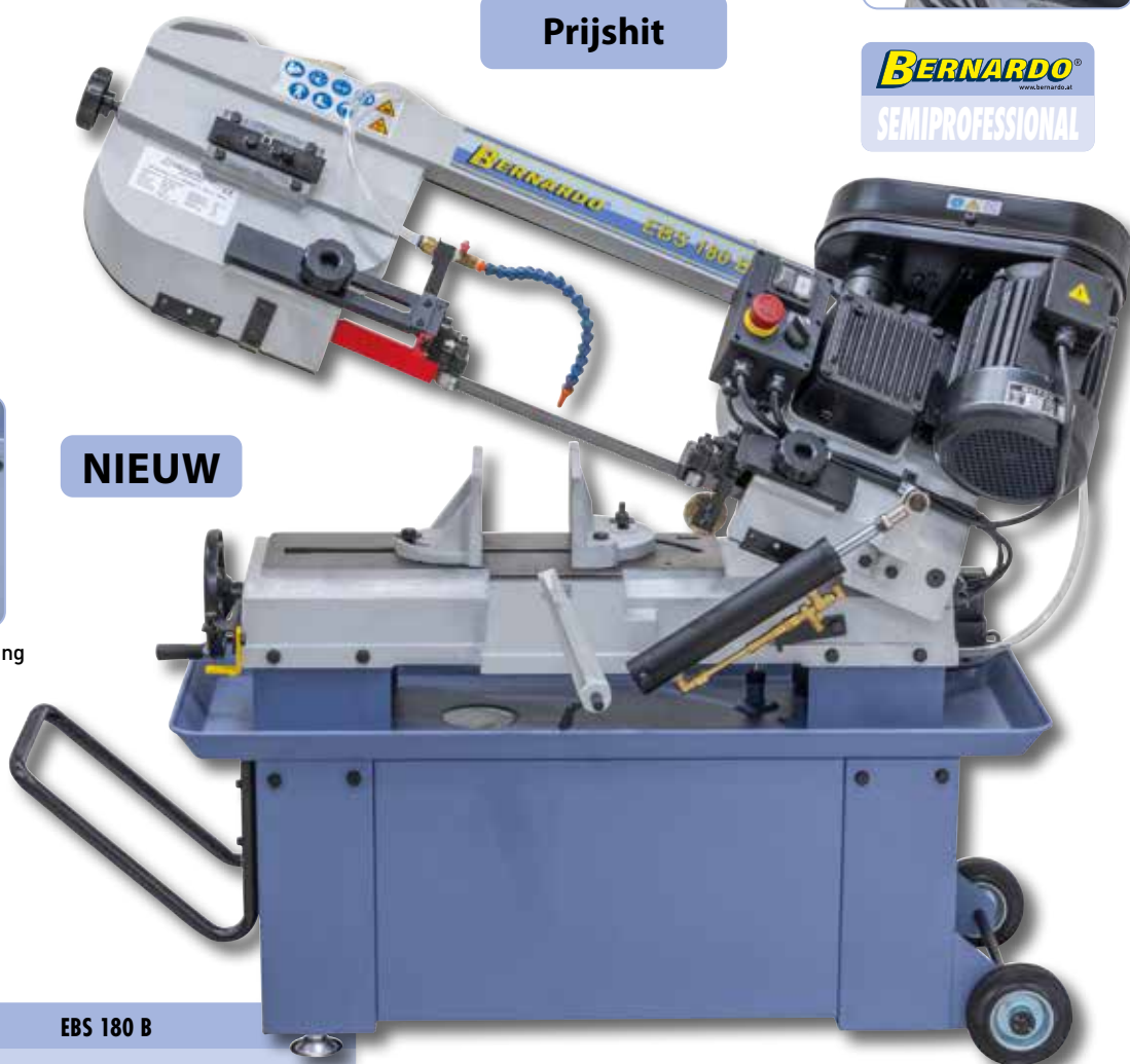
Groot bemeten hydraulische cilinder voor traploze neerlaat van de zaagbeugel
