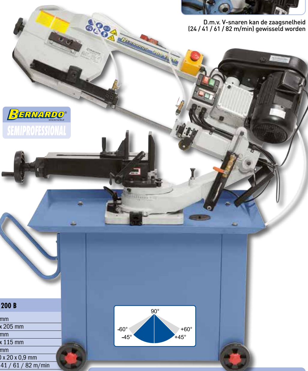
Zwenkbare zaagbeugel voor verstekzagen van -45^\circ tot +45^\circ verstelbaar
