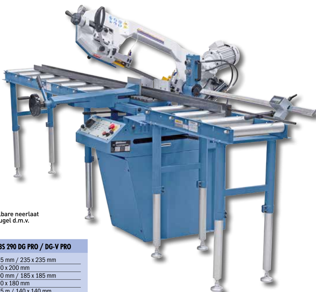
Gecombineerde rollen en hardmetalen geleiding voorkomt snel verslijten van de zaagband.
