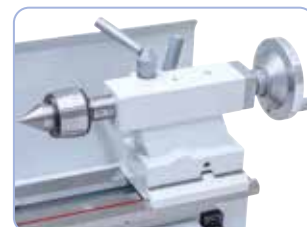
Nyeregszege MK 2 felvétellel kúpesztergáláshoz beállítható
