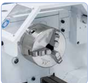
3-pofás tokmány 125 mm, eszterga- és fúrópofákkal a szállítási terjedelemben
