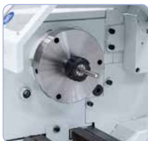
A szorítófogó-tokmány ER 25 a körmozgás nagy pontosságát biztosítja munkadarabok befogásánál, befogási tartomány 1 - 16 mm
