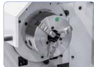
A Bernardo-pofás tokmány előnye DK11-200 mm / D5: Monoblokk-, alap-, fordító- és feltépfókával szállítható
