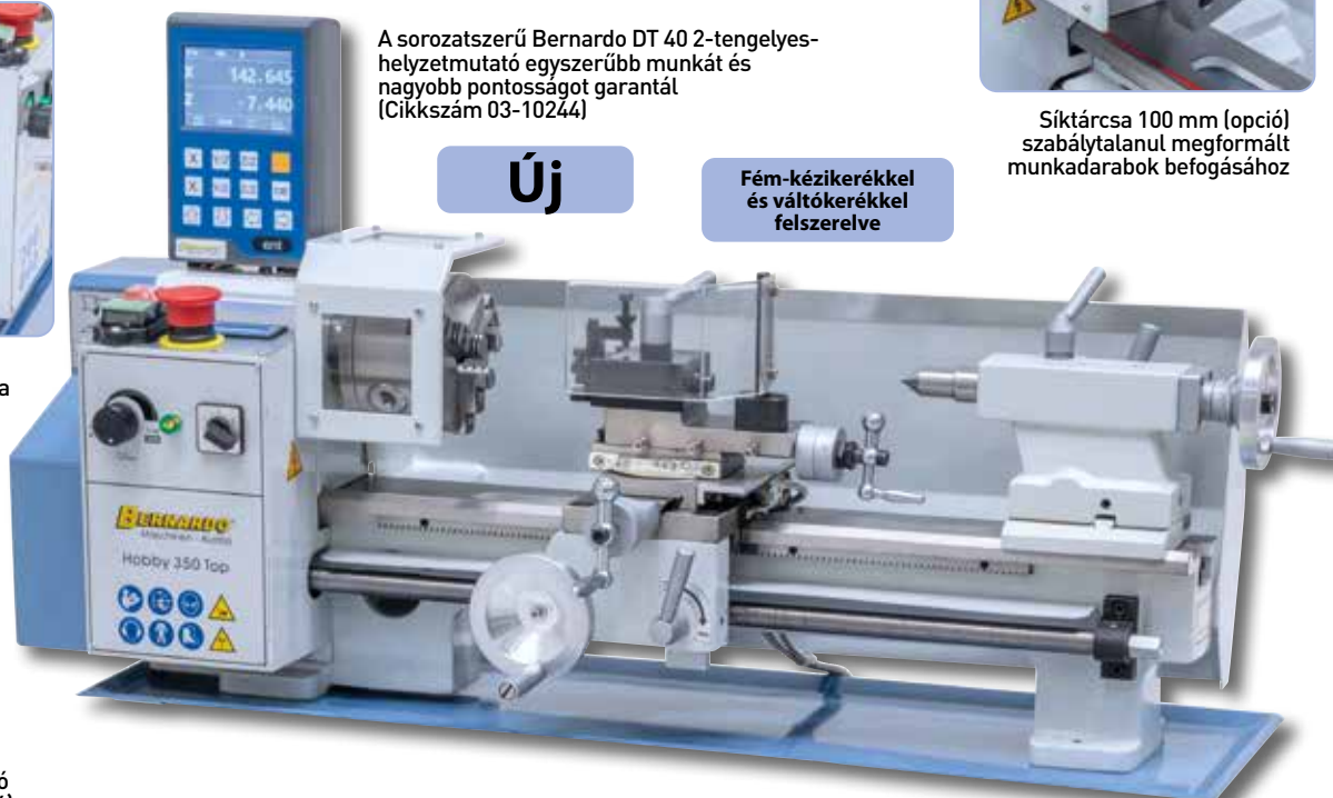
Sorozatszerűen acél váltókerekkel menetvágáshoz a szállítási terjedelemben
