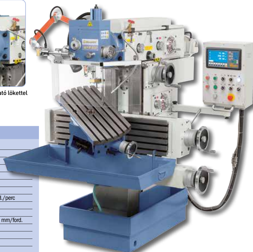
Függőleges befogási felület 5 T-horonnyal az univerzális billenőasztal (opció), ill. a szilárd szög.asztal egyéni befogásához
