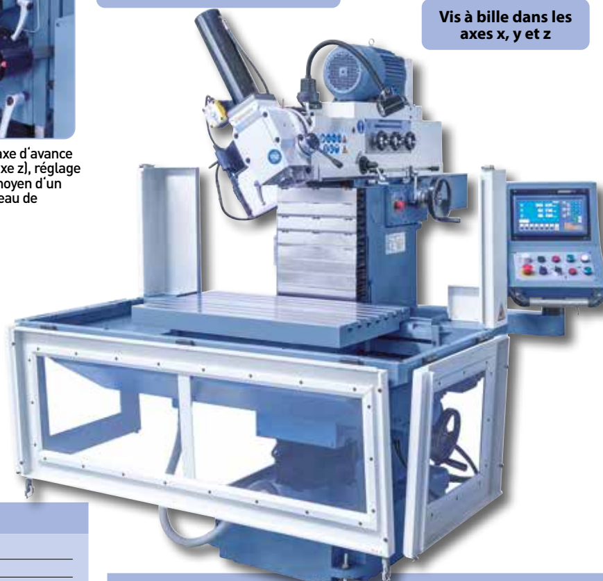
Éléments de commutation disposés clairement sur le pupitre de commande pivotant, de série avec affichage numérique à 3 axes à écran LED..
