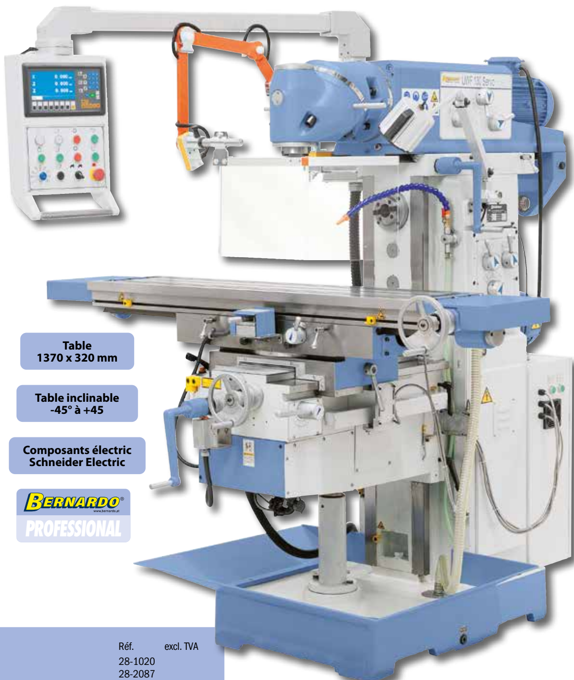
Le grand guide rectangulaire sur les axes y et z garantit une stabilité accrue
