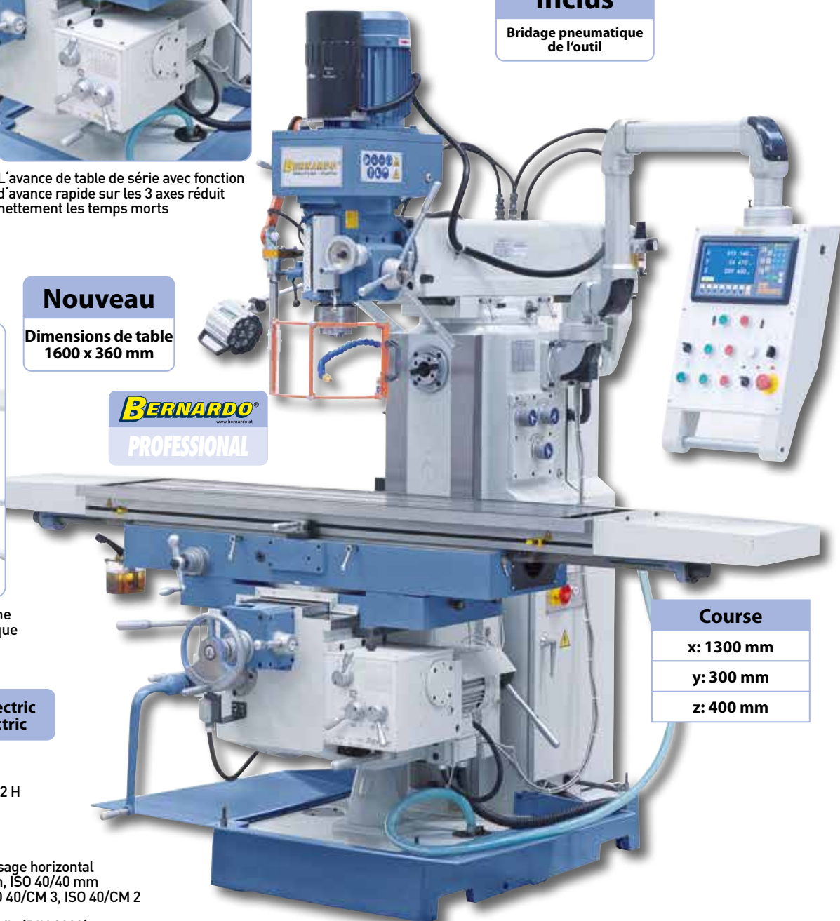
Pupitre de commande parfaitement lisible et accessible. Visu dynamique de série
