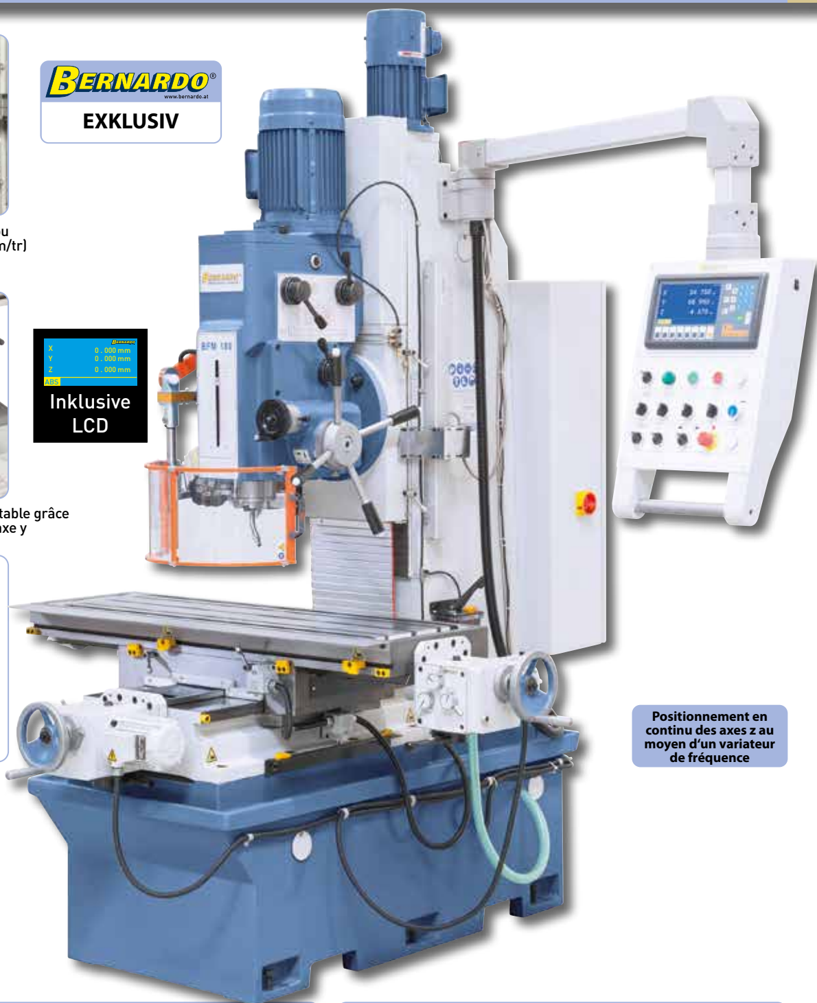
Réglage de la table sur l'axe x au moyen de 8 vitesses d'avance au choix (24 - 720 mm/min)
