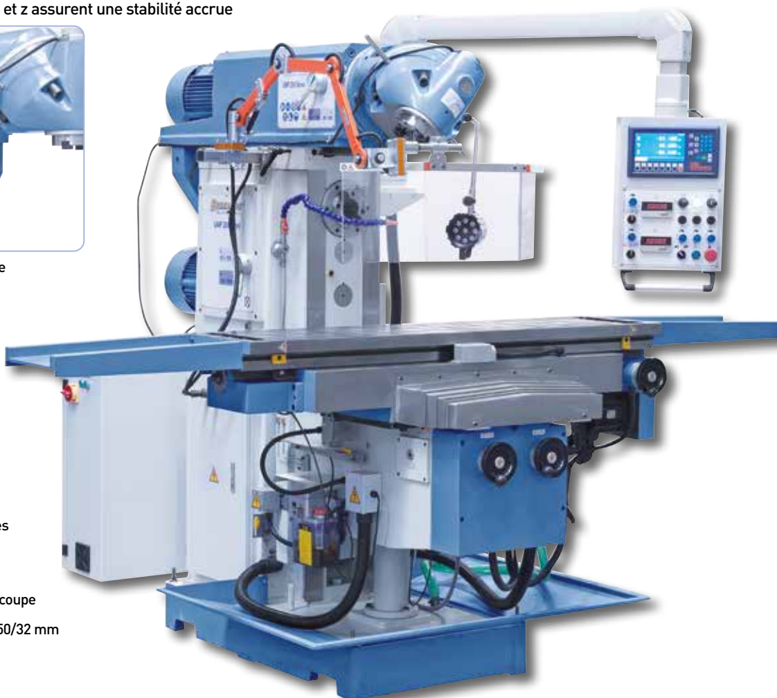
De série avec contre-broche et longue broche pour le fraisage horizontal
