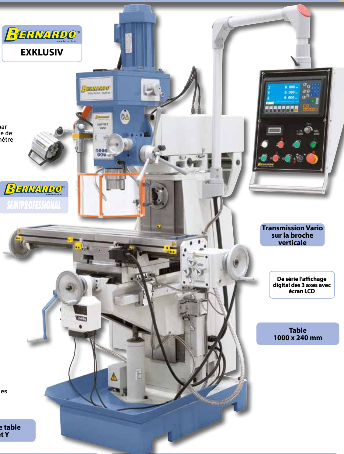
Descente et montée de broche par levier, ajustement de précision par manivelle
