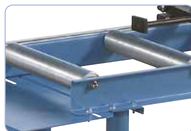
Teräsrollissa on kuulalaakerit molemmilla puolilla – tarkoitettu raskaille kuormille
