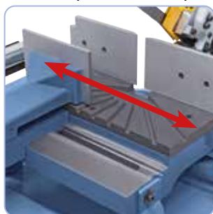
Pikalukituksella varustettu ruuvipuristin on käännettävissä kaksoisviistesahauksia varten
