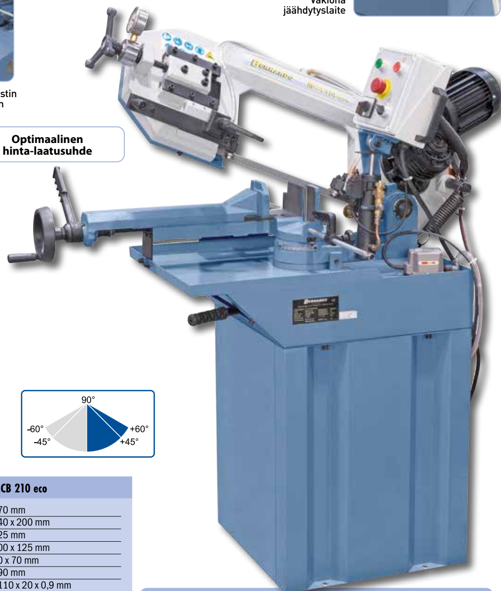
Vakiona jäähdytyslaite
