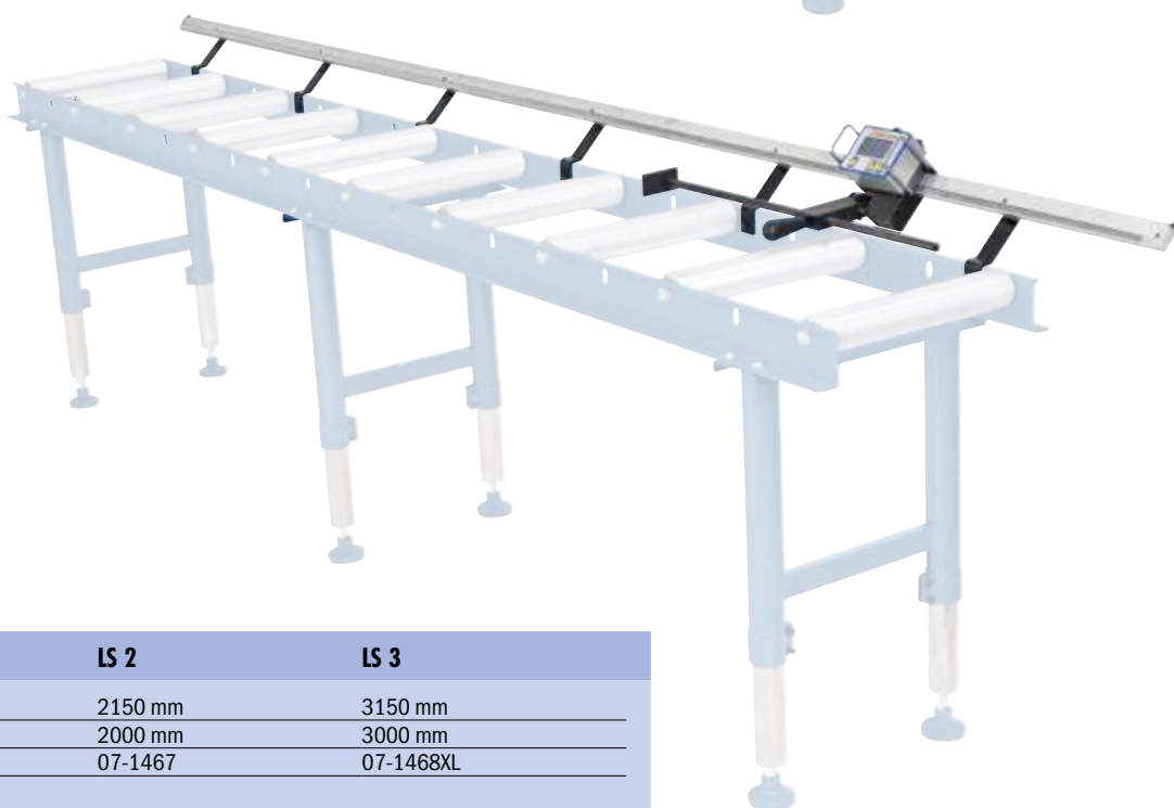
Ylöstaitettava materiaalivaste, voidaan käyttää joko oikealla tai vasemmalla
