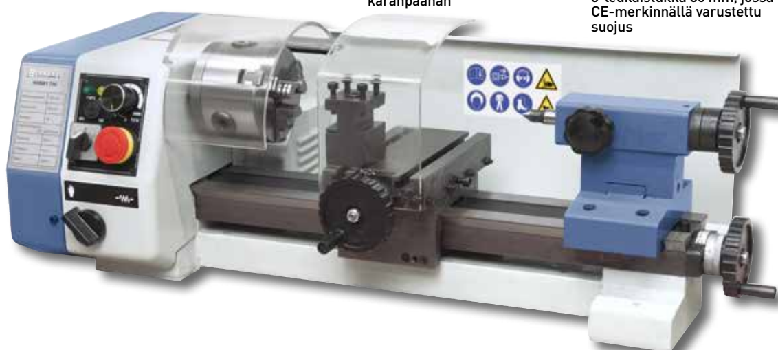
Helppokäyttöinen, kaikki kytkimet sijoitettu karanpäähän
