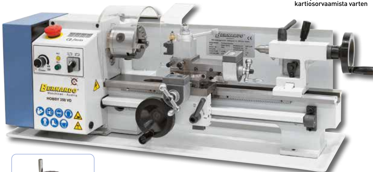
Takapylkkä, jossa MK 2 kiinnitys, voidaan muuttaa kartiosorvaamista varten
