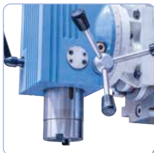
Suurikokoinen kara (Ø 90 mm) takaa parhaan mahdollisen vakauden
