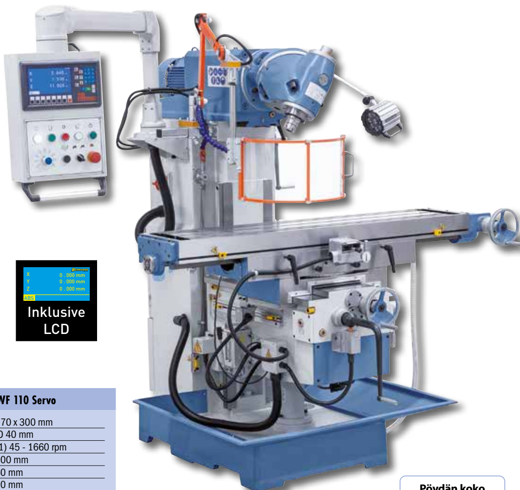
Vakiona vastalaakeri ja pitkä jyrsintuurna vaakajyrsintään.
