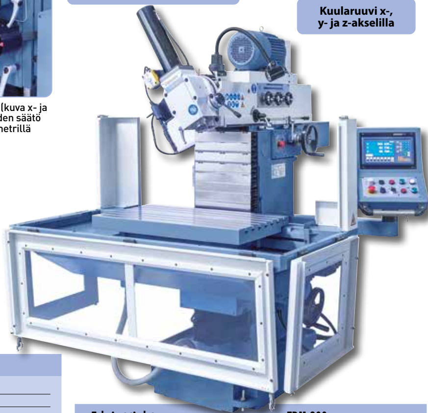
Sis. hydraulinen työkalukiinnike vetokaralla (DIN 69872)
