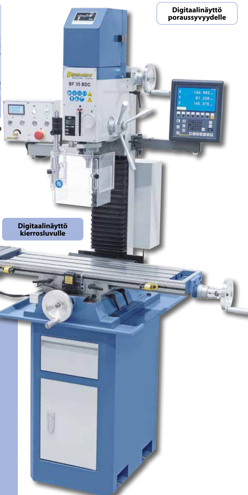
Molemminpuolisesti kallistettava jyrsinpää -90° - +90°
