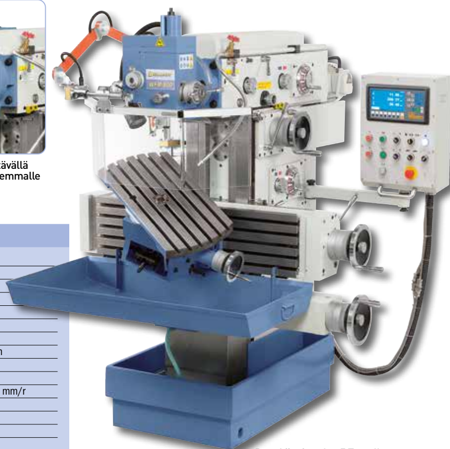
Pystykiinnitysalue 5 T-uralla yksittäiskiinnitykseen lisävarusteena saatavana kääntyvä yleisjyrsinpöytä tai vakio työpöytä.
