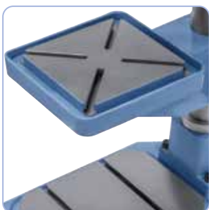
Hiottu työpöytä, jossa samansuuntaisesti kulkevat T-urat.
