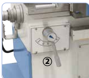
1: Håndtag til fremføringsretning 2: Håndtag til fremføringsakse
