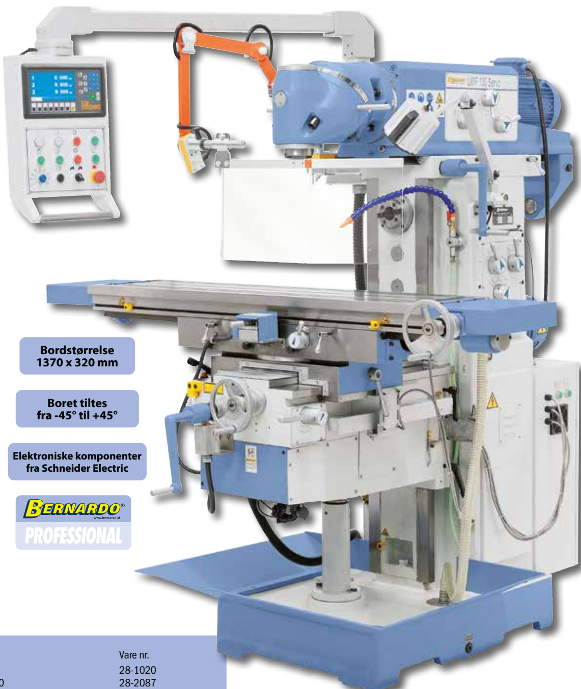
Universalfræsehoved med 2 drejaksler, justerbart til alle vinkelpositioner.
