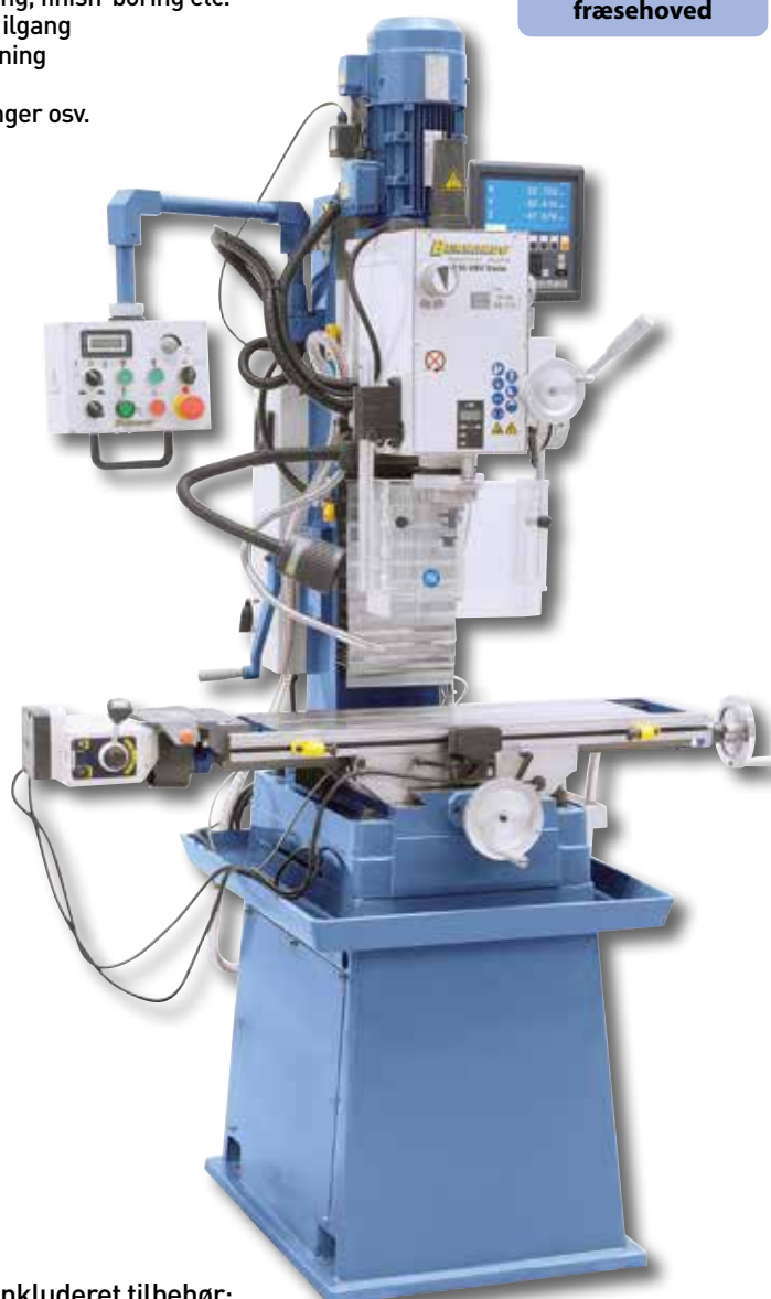
Stort krydsbord med T-notsport og kølemiddel-fordybning. Billede med valgfri fræsebords-fremføring AL 450 D
