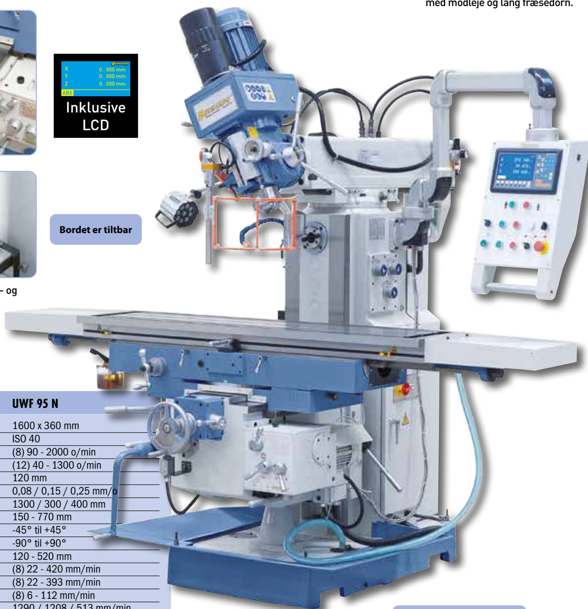
Til fræsning i vandret position med modleje og lang fræsedorn.
