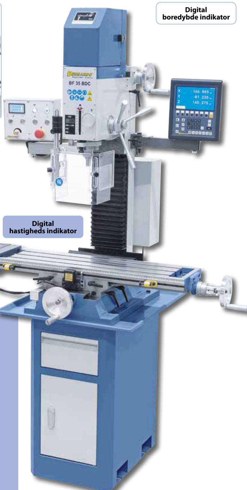
Fræsehoved kan tiltes til begge sider fra -90 ° til +90 °.
