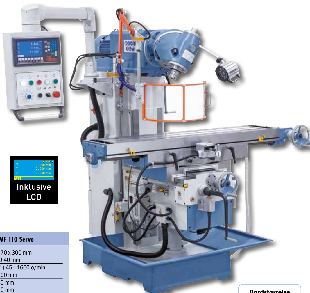
Enkelt betjening af betjeningsselement til skift af omdrejningstal.
